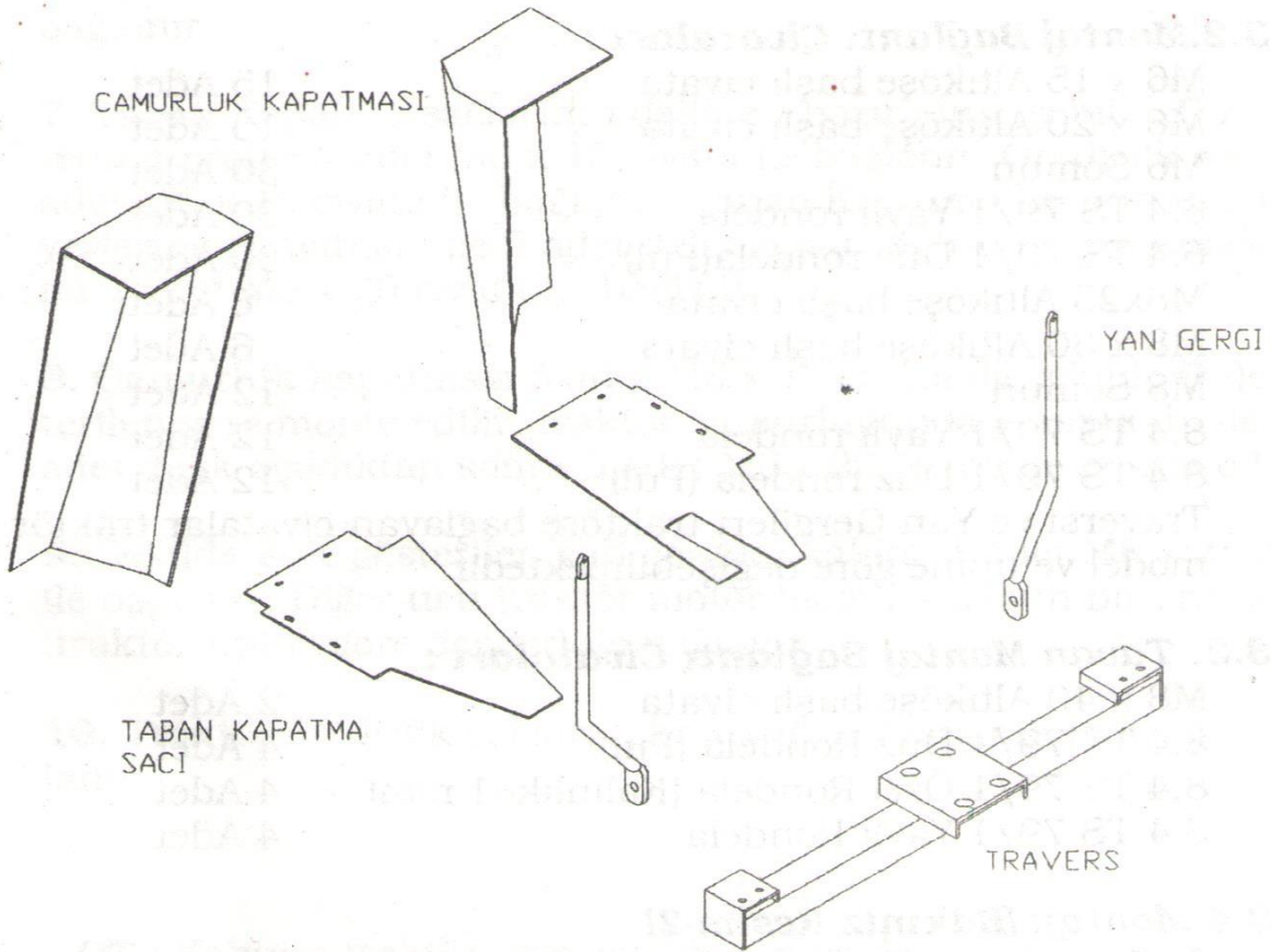
Resim-1. MONTAJ PARÇALARI
