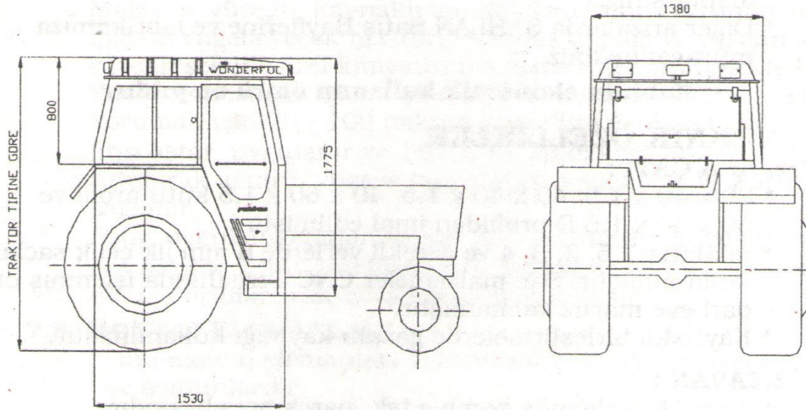
Resim-10 KABİNİN GENEL BOYUTLARI
