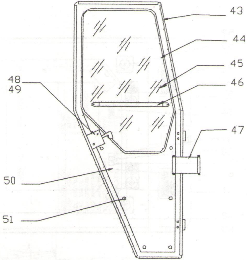
Resim-6 KAPI İÇ GÖRÜNÜŞÜ
