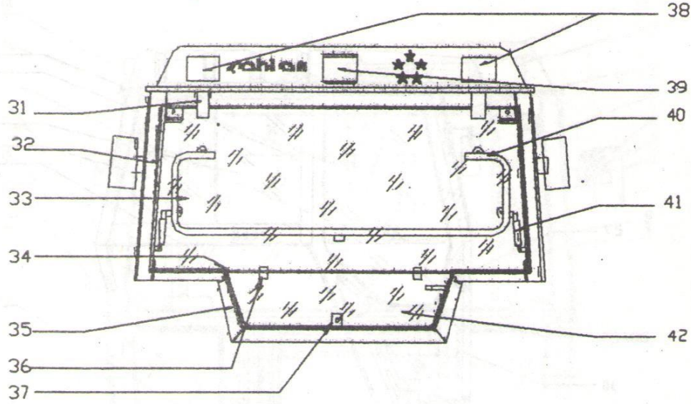
Resim-5 KABİNİN ARKADAN GÖRÜNÜŞÜ
