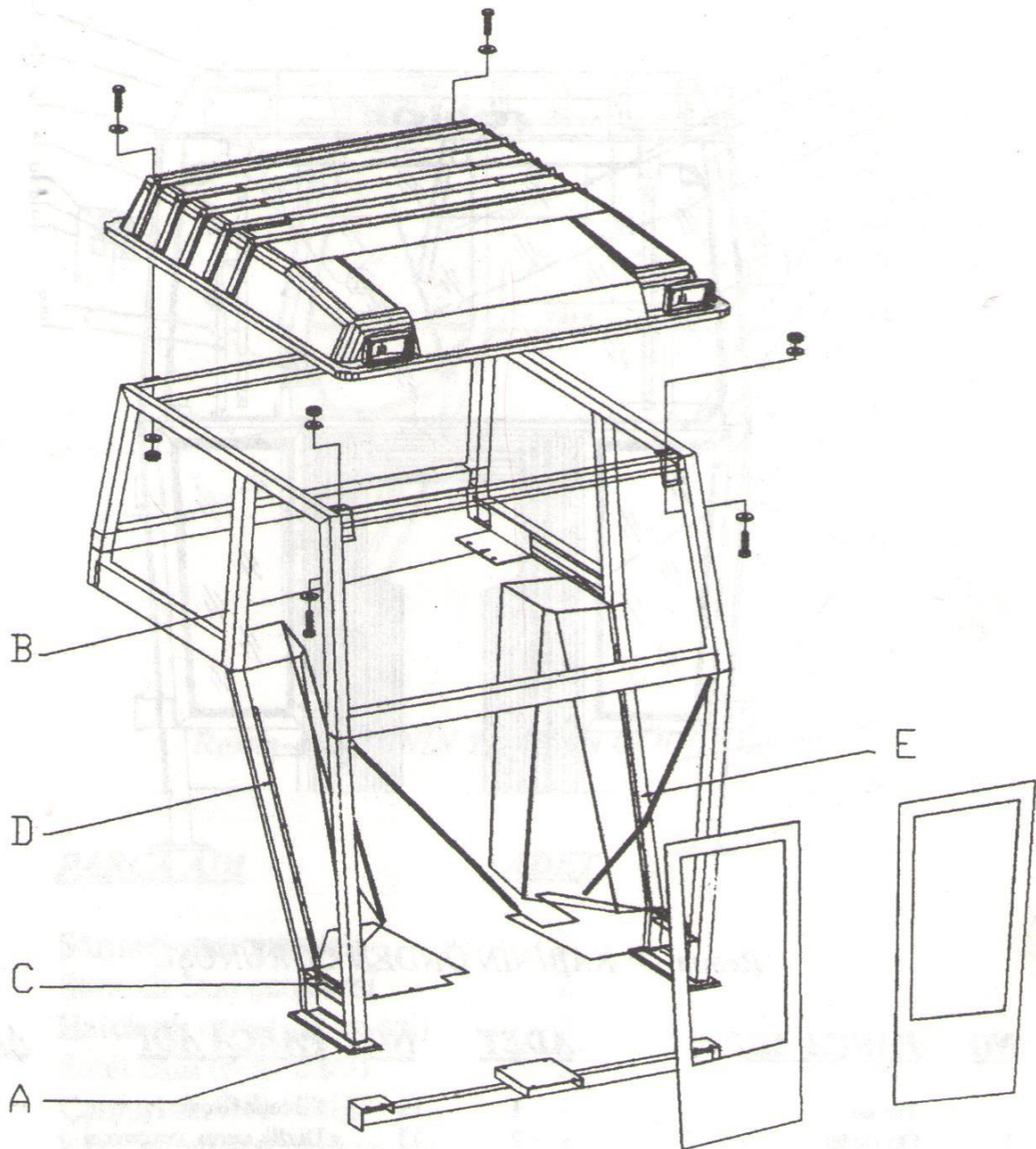
RESIM-2. KABININ PERSPEKTIF GORUNUSU
