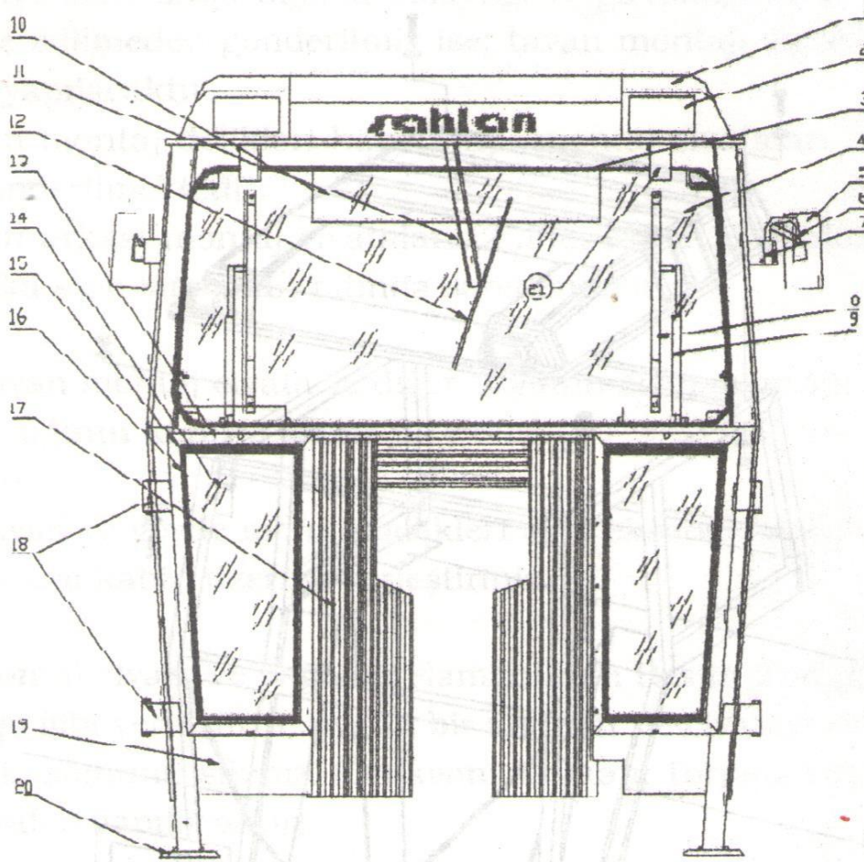
Resim -3: KABİNİN ÖNDEN GÖRÜNÜŞÜ
