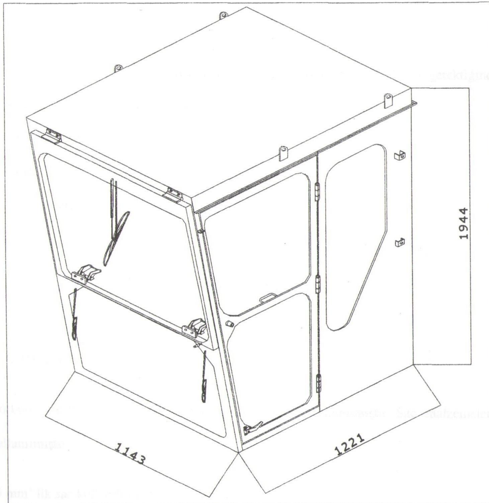
Resim 7: KABİNİN GENEL BOYUTLARI
