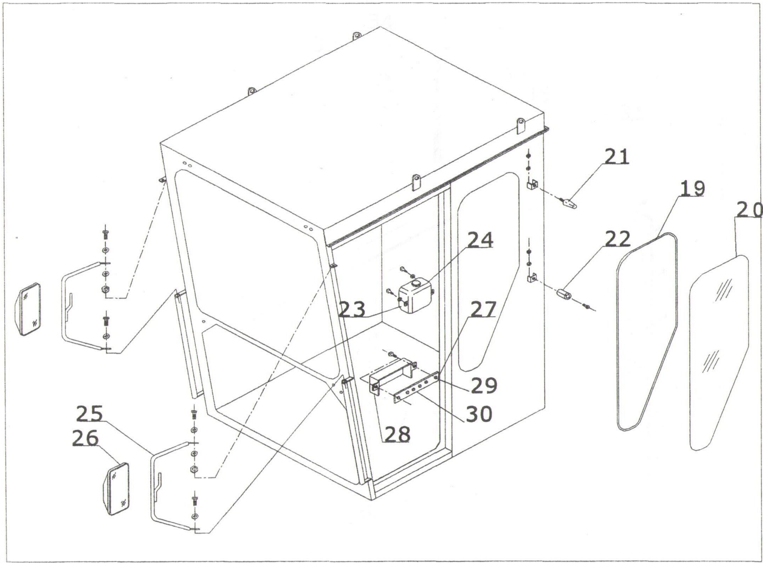
Resim -3: KABİNİN YANDAN GÖRÜNÜŞÜ
