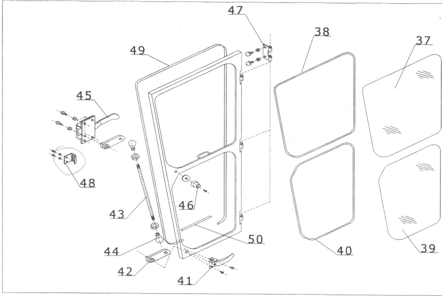
Resim-5 KAPI İÇ GÖRÜNÜŞÜ
