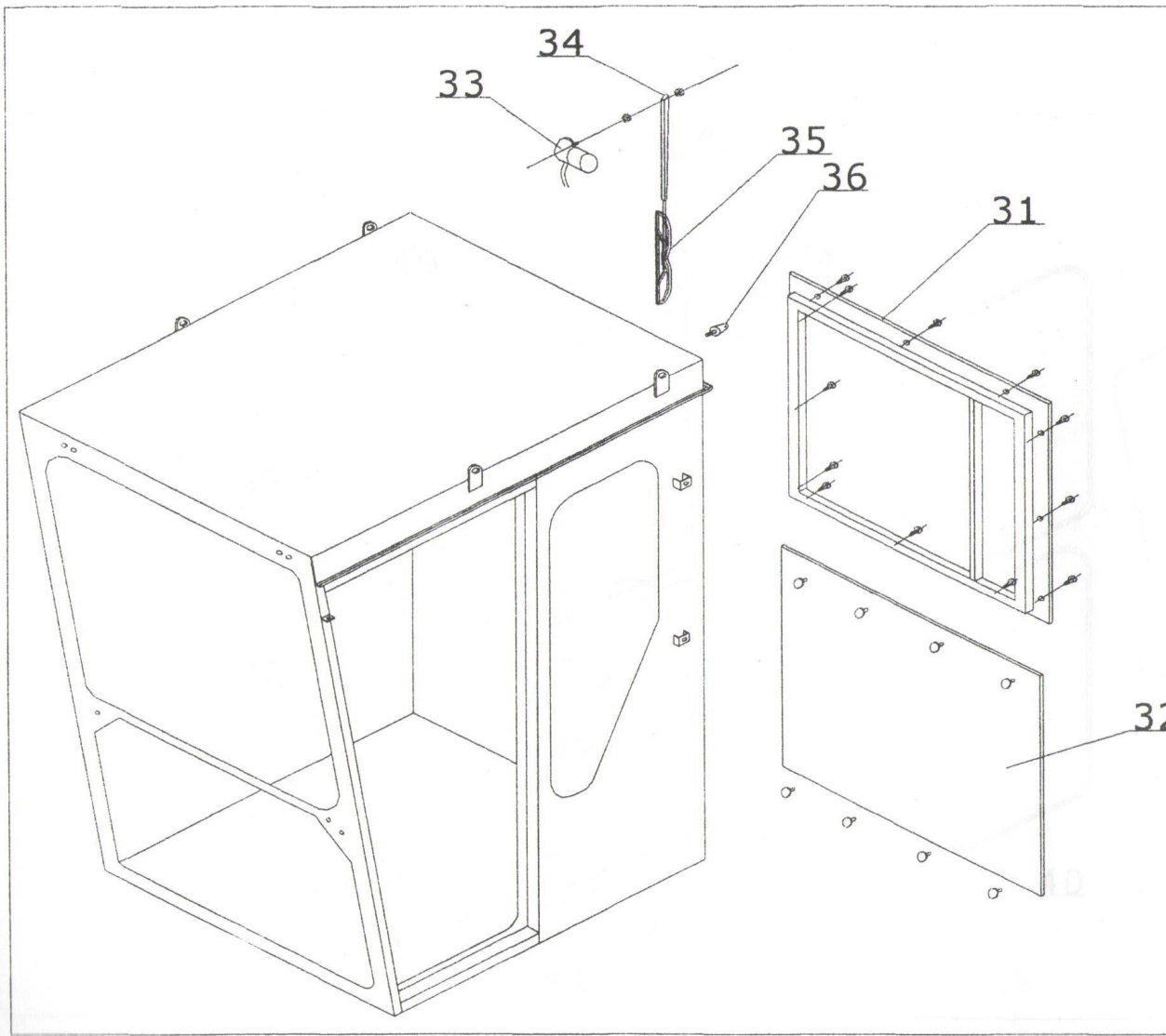
Resim-4 KABİNİN ARKADAN GÖRÜNÜŞÜ
