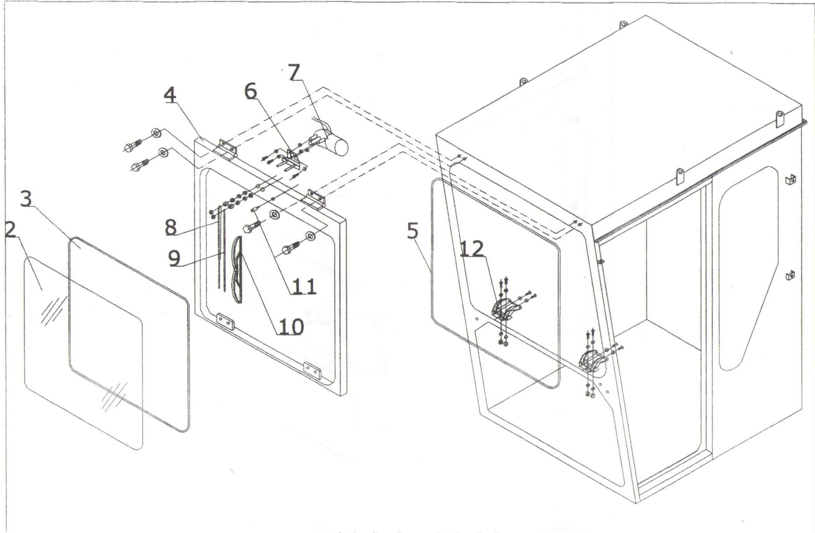
Resim 1: KABİNİN ÖN ÜST GÖRÜNÜŞÜ
