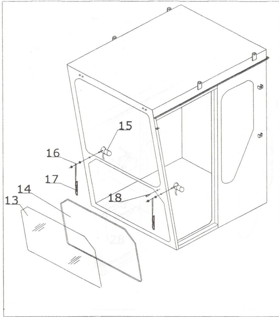
Resim -2: KABİNİN ÖN ALT GÖRÜNÜŞÜ
